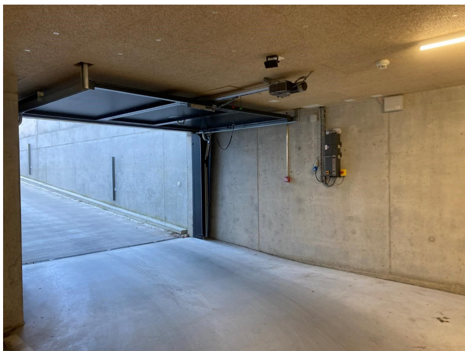
Einstellhallen-Kipptor ET500 mit Schlupftüre Innenansicht (Tor offen)
